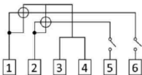
Medidor com relé interno
